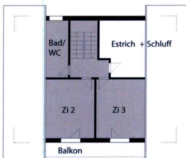
Dachgeschoss
