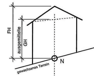
Ausgemittelte Gebäudehöhe
