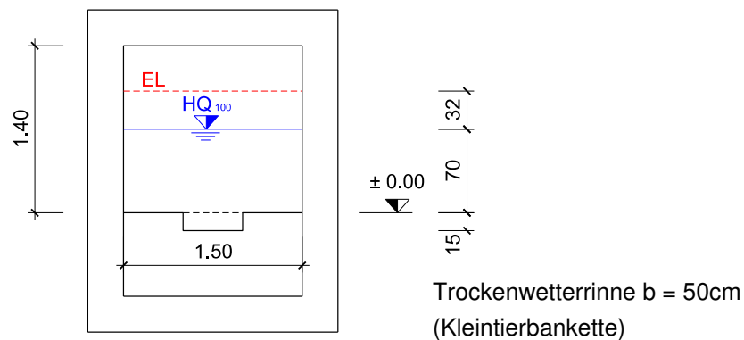
Abbildung 2: Gewählter Querschnitt (Durchlass)
