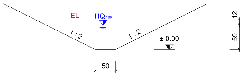
Abbildung 3: Gewählter Bachquerschnitt (Trapezprofil)
