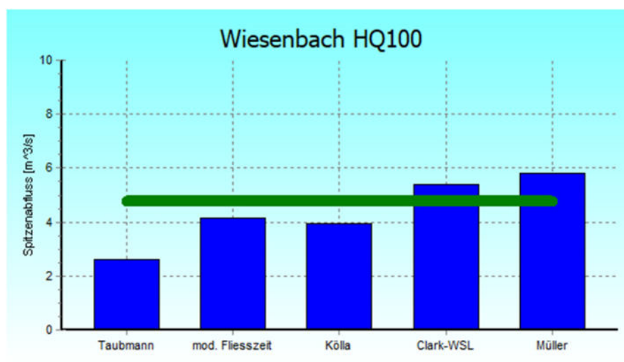
Abbildung 3: Grafik Resultate Ermittlung Wiesenbach, Vorschlag HAKESCH
