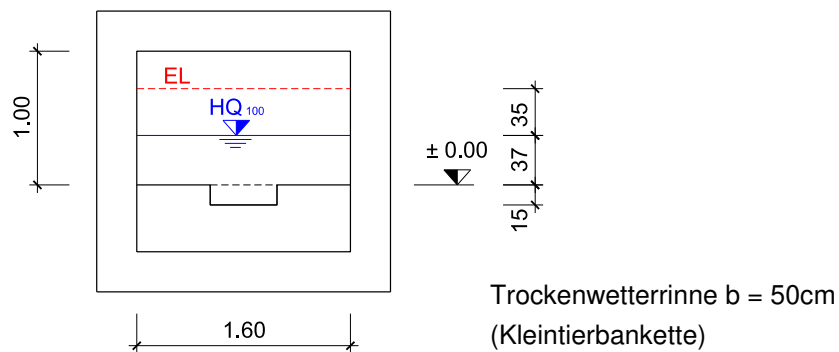
Abbildung 4: Gewählter Querschnitt (Durchlass)
