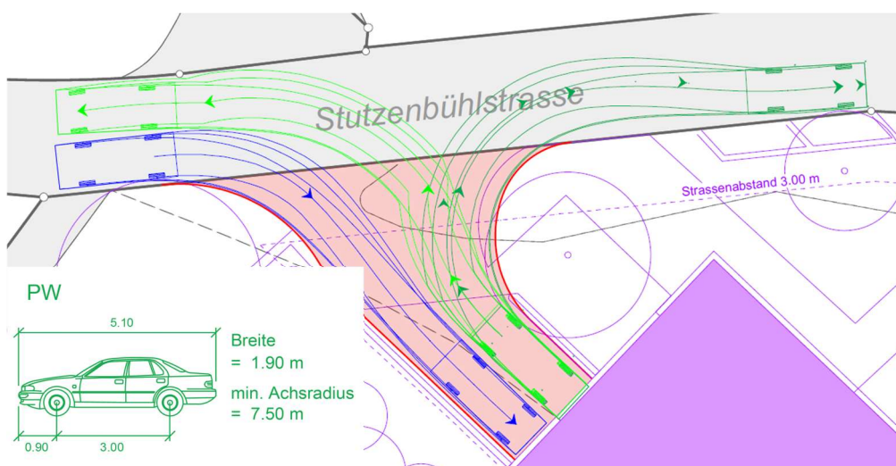
Abbildung 18: Schleppkurven- überprüfung
