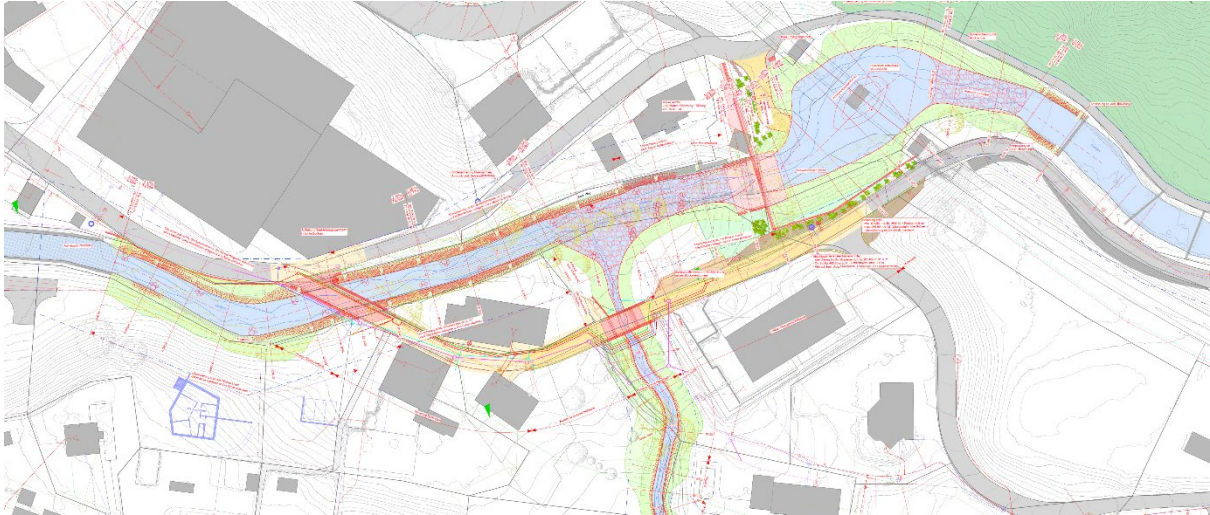
Abb. 7: Plan, Wasserbauliche Vorstudie
