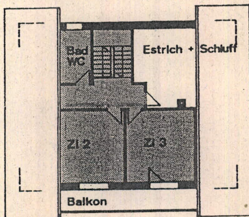
Dachgeschoss
