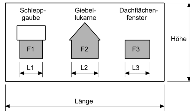
Ansicht Dachfläche
